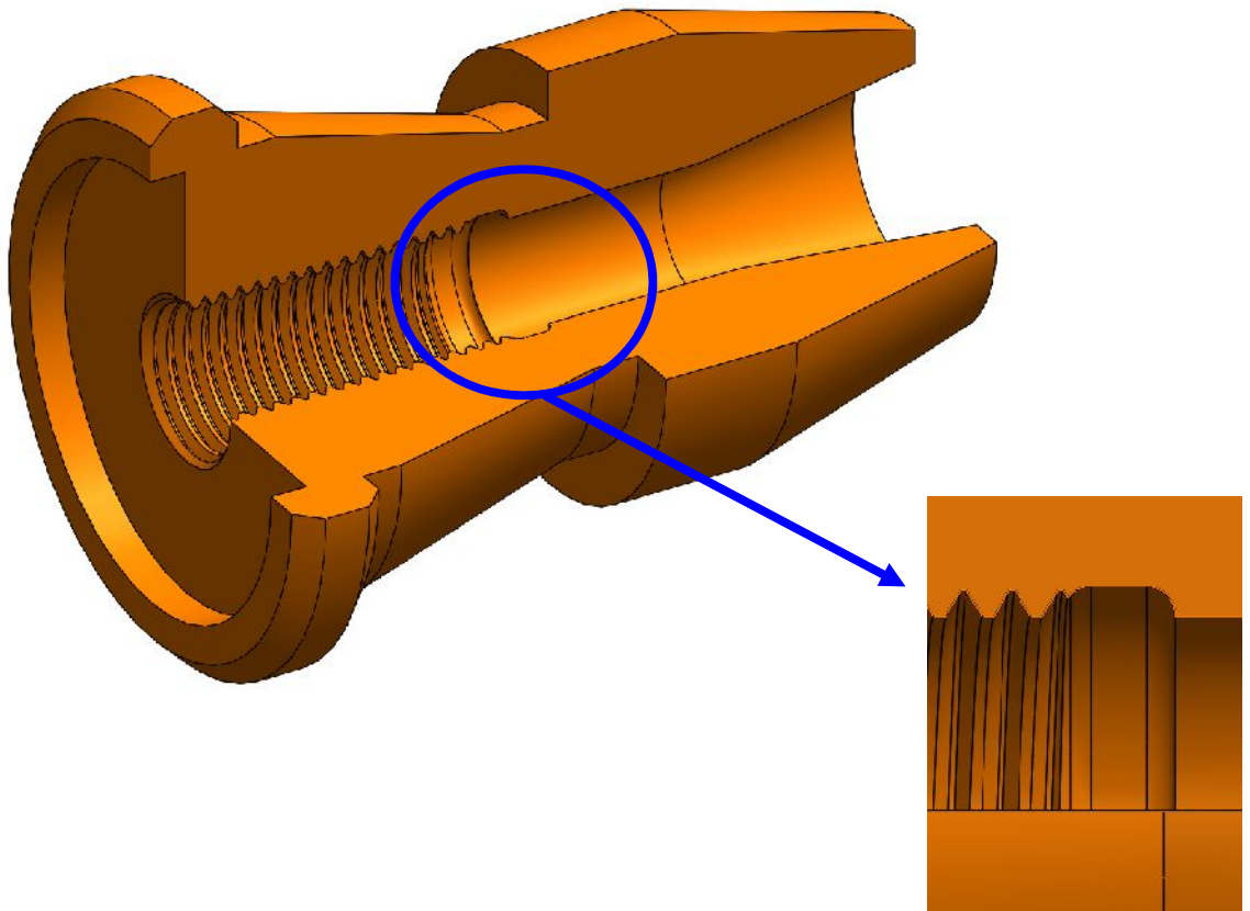
Rez hriadel'om
